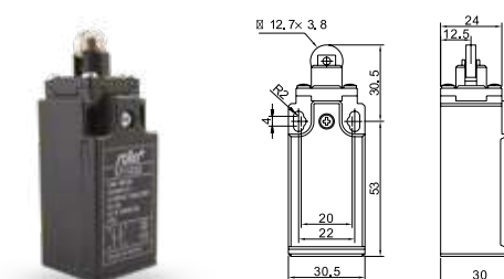
STI 1032 - Görgős végálláskapcsoló / Roller plunger type
