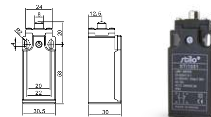
STI 1031 - Bútykós végálláskapcsoló / Push plunger type
