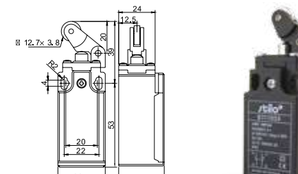
STI 1033 - Egyirányú vízszintes működtetésű görgős végálláskapcsoló / Horizontal roller lever type
