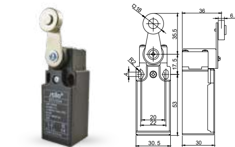
STI 1034 - Karos-görgős végálláskapcsoló / Roller arm type
