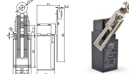
STI 1035 - Állítható karos-görgős végálláskapcsoló / Adjustable roller arm type
