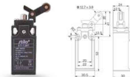
STI 1381 - Egyirányú, függőleges működtetésű görgős végálláskapcsoló / Vertical roller lever type
