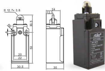
STI 1032 - Görgős végálláskapcsoló / Roller plunger type
