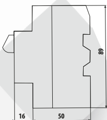
Méreték /Size (mm)
