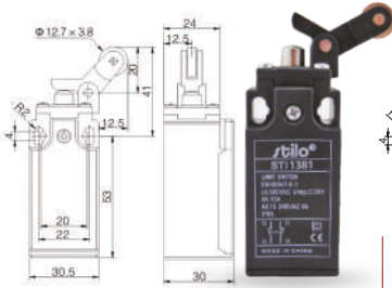
STI 1381 - Egyirányú, függőleges működtetésű görgős végálláskapcsoló / Vertical roller lever type
