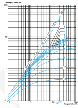
Áramkorlátozási jelleggörbe / Current limit characteristic
