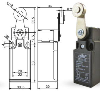
STI 1034 - Karos-görgős végálláskapcsoló / Roller arm type
