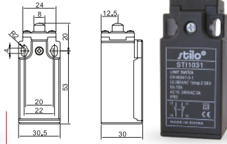
STI 1031 - Büttykös végálláskapcsoló / Push plunger type
