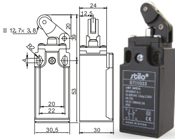
STI 1033 - Egyirányú vízszintes működtetésű görgős végálláskapcsoló / Horizontal roller lever type
